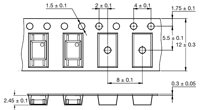
Fig. 18 - Tape Dimensions
