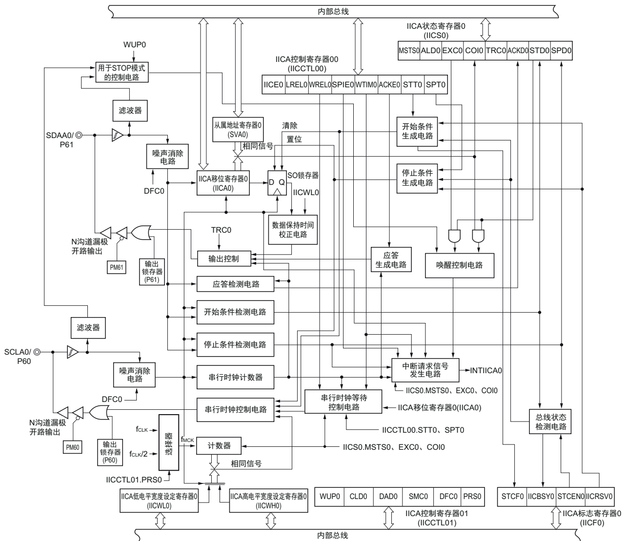
图 12-1 串行接口 IICA 的框图
