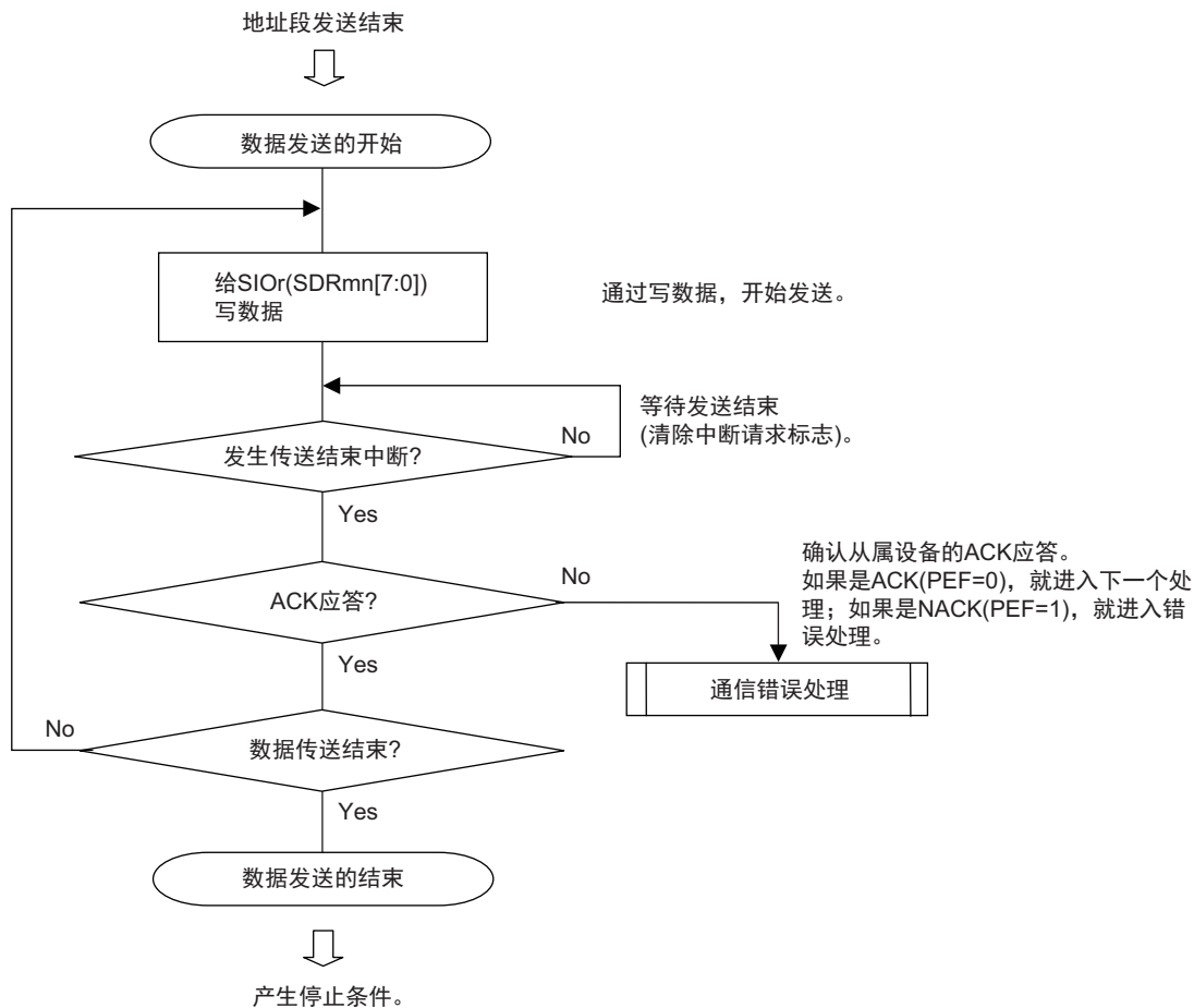
图 11-103 数据发送的流程图
