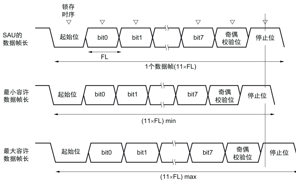
图 11-94 接收时的波特率容许范围 (1 个数据帧的帧长 = 11 位的情况)
