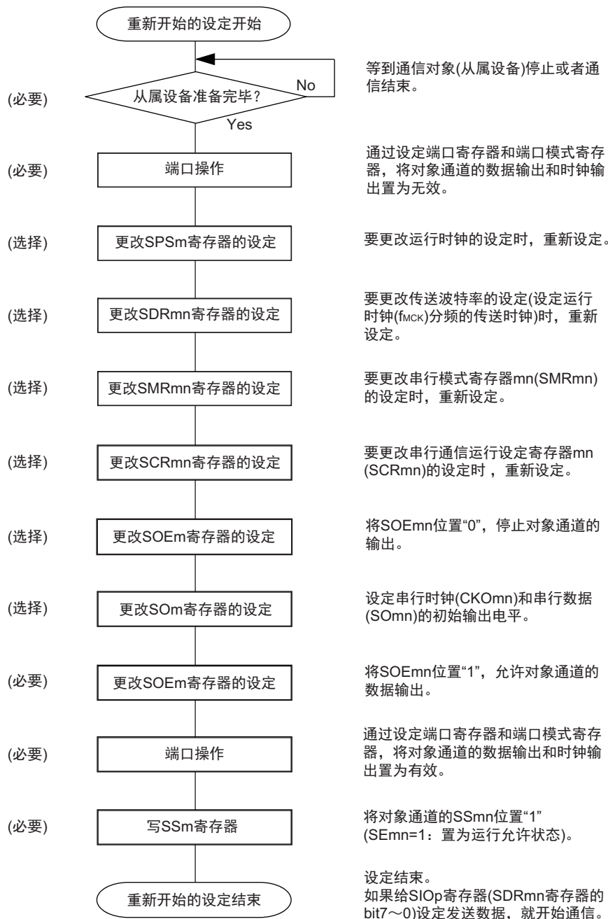
图 11-27 重新开始主控发送的设定步骤
