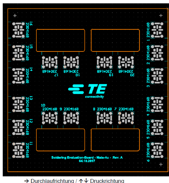
Figure / Bild 7: Soldering Test PCB / Platine für Löttest
