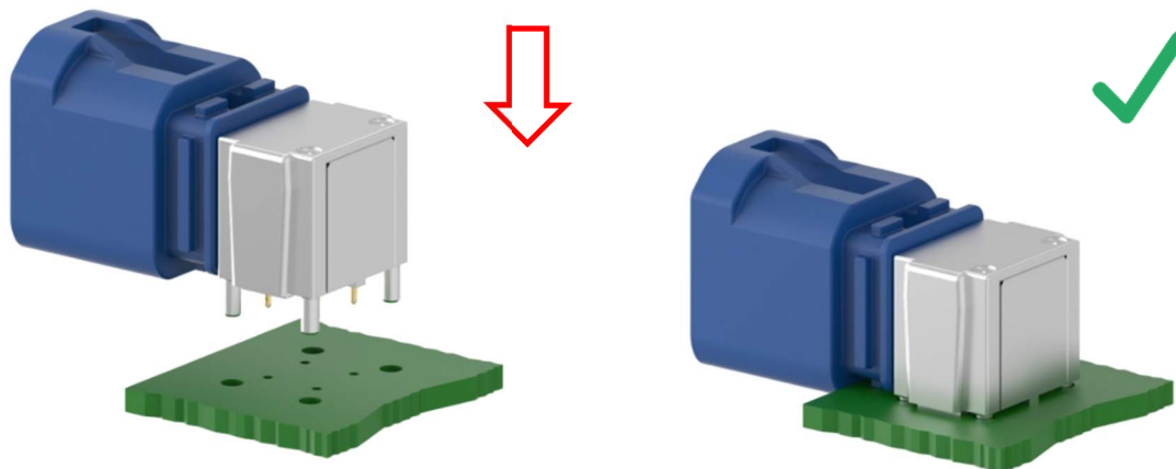
Figure 2 / Bild 2: MATE-AX 4 pos. Header / MATE-AX 4 pol. Stiftwanne Geometry shown in simplified view/ Geometrie vereinfacht dargestellt
