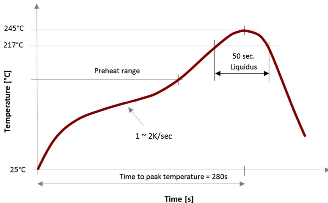
Figure / Bild 6: Temperatur-Time Profile / Temperatur-Zeit-Profil
