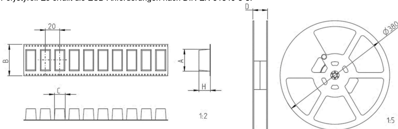
Figure / Bild 1: Packaging Dimensions [mm] / Verpackungsmaße [mm]
