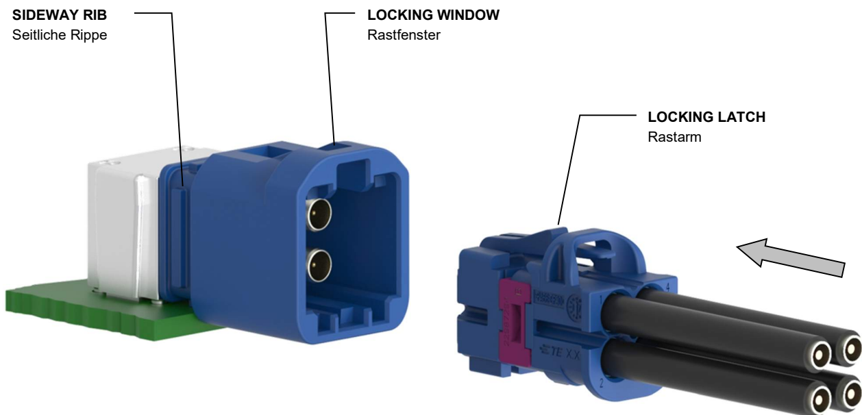
Figure / Bild 8: Assembly with cable connector / Montage mit Kabelbaumsteckverbinder
